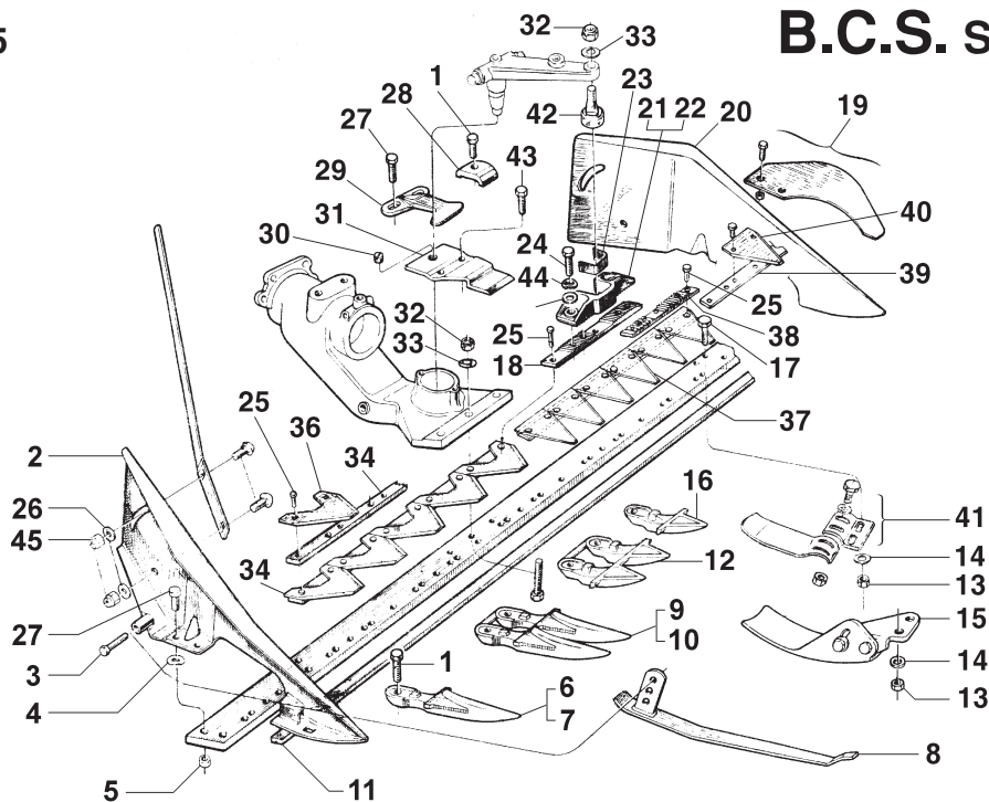
RICAMBI ADATTABILI A: B.C.S. SERIE 600 - 700
